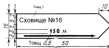
Рис.2 Показчик маршруту руху до захисної споруди
